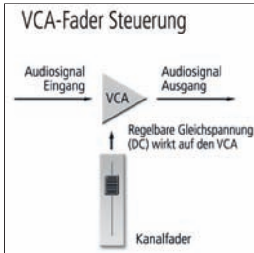
... und hier könnt ihr den Signalfluss sehen, wie er bei einer VCA-Gruppe stattfindet.
